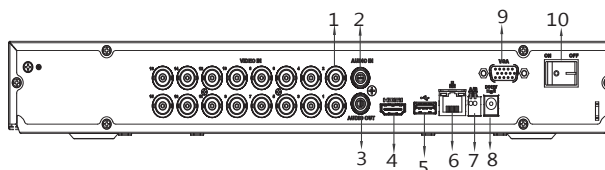
DH-XVR5216AN-4KL-X
