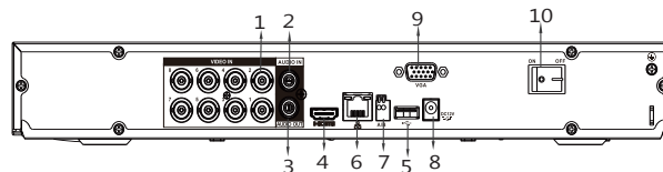
DH-XVR5208AN-4KL-X
